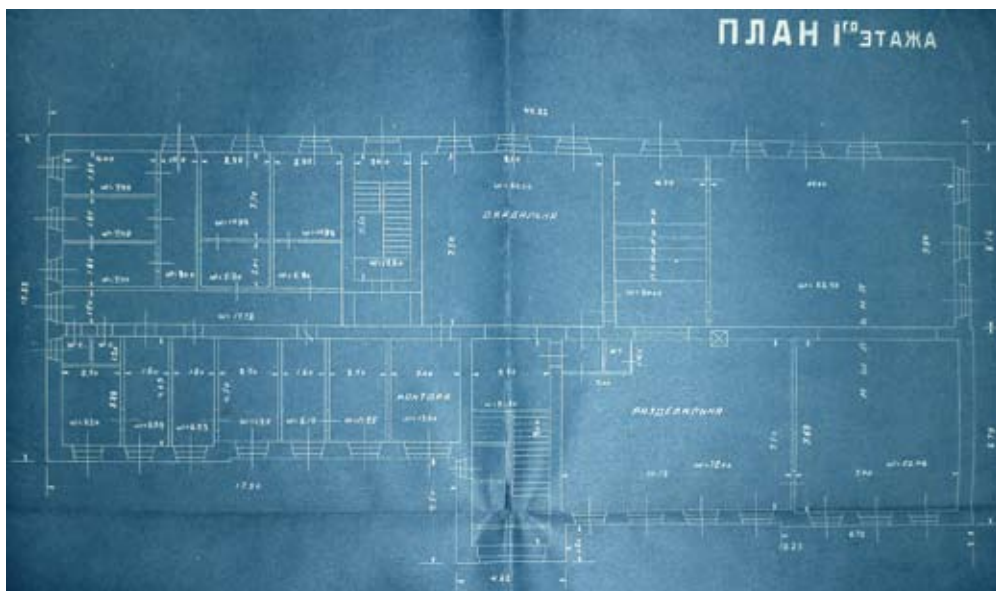
Рис. 23. Проект коммунальной бани в Красноярске. План 1-го этажа (1929) [18]
