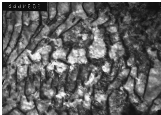
Рис. 3. Структура стали марки 80Р с УМЗ после МТО 400 °С/58 800 Н (светлопольное изображение, увеличение 50 000)
