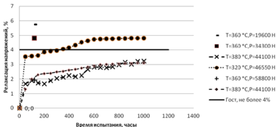
Рис. 4. Релаксация напряжений высокопрочной арматуры из стали марки 80Р после МТО с различными значениями параметров процесса
