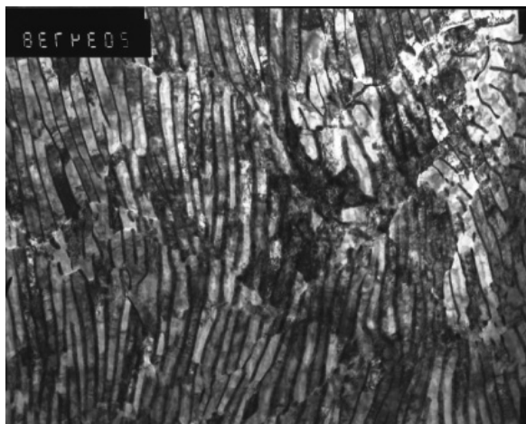
Рис. 2. Структура стали марки 80Р после МТО 360 °С/46 600 Н (светлопольное изображение, увеличение 20 000)
